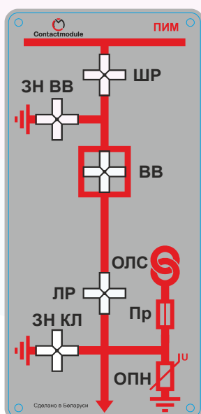
ПАНЕЛЬ ИНДИКАЦИИ МНЕМОСХЕМЫ
